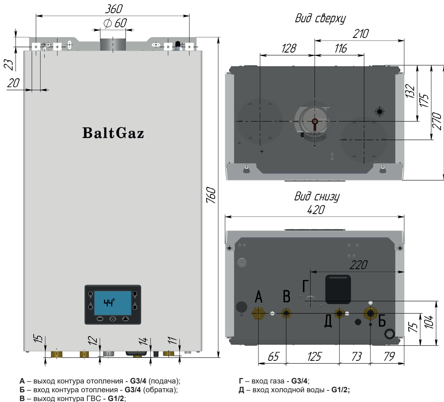
Рис. 1 Габаритные и присоединительные размеры котлов
